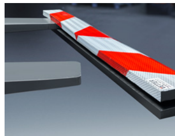
Magnetische Einfahrtaschen (KEINE Bearbeitung der Gabelzinken notwendig)
