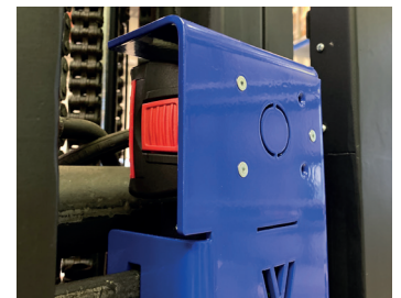
Kabellose Energieversorgung mit VETTER SmartSupply
